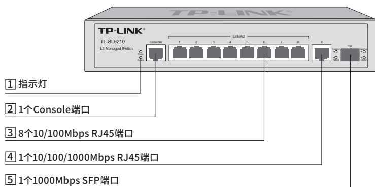
图1-16 TL-SL5210前面板示意图
